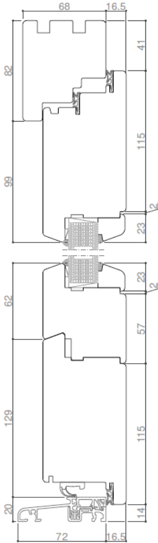
Haustür mit Schwelle nach innen öffnend
