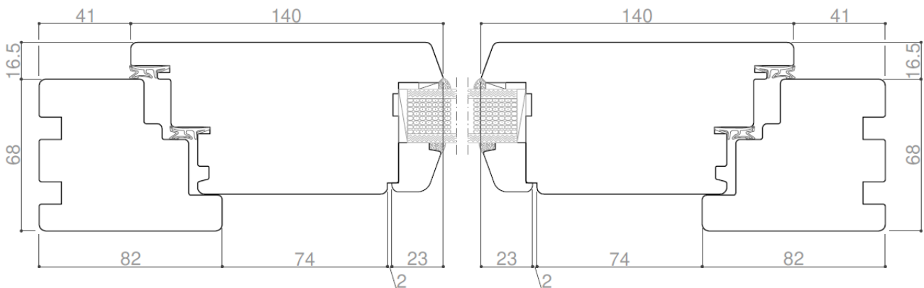
Haustür nach außen öffnend
