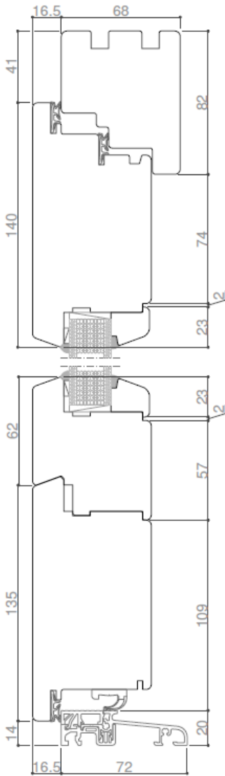
Haustür mit Schwelle nach außen öffnend
