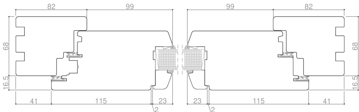
Haustür nach innen öffnend
