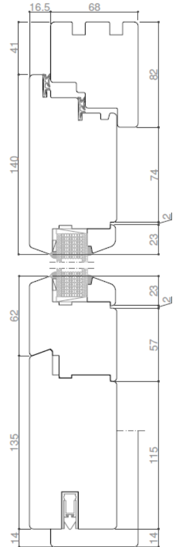
Haustür mit Kältefeind nach außen öffnend
