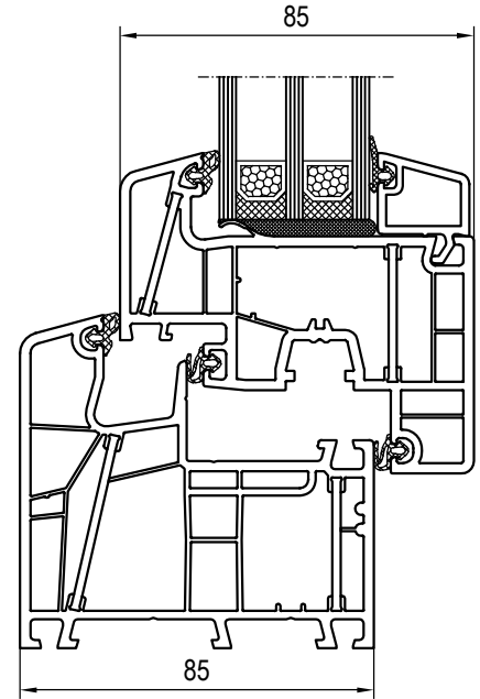
Zugrundeliegende Profil-Kombination für U_f Maßstab: 1:2
